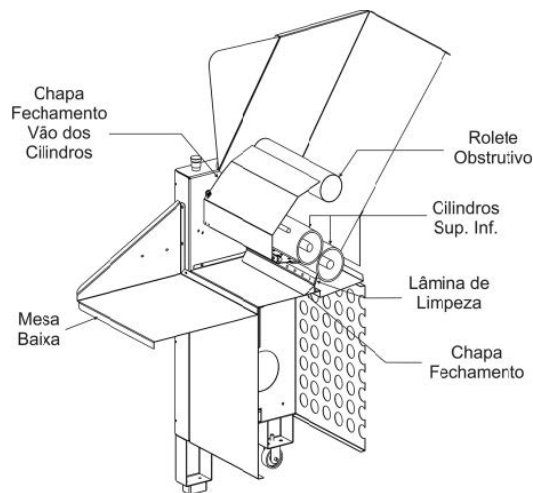
Figura 1: Representação esquemática do cilindro soador.
